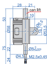
2138-10 2139-10
