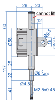
2138-25 2139-25
