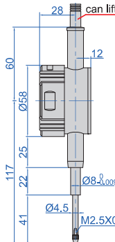
2138-25P 2139-25P
